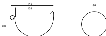
Regenwaterafvoersysteem 125/88 mm
